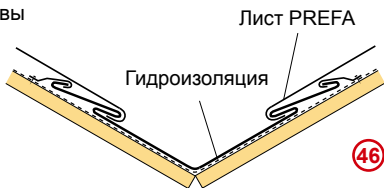
Вариант монтажа ендовы
